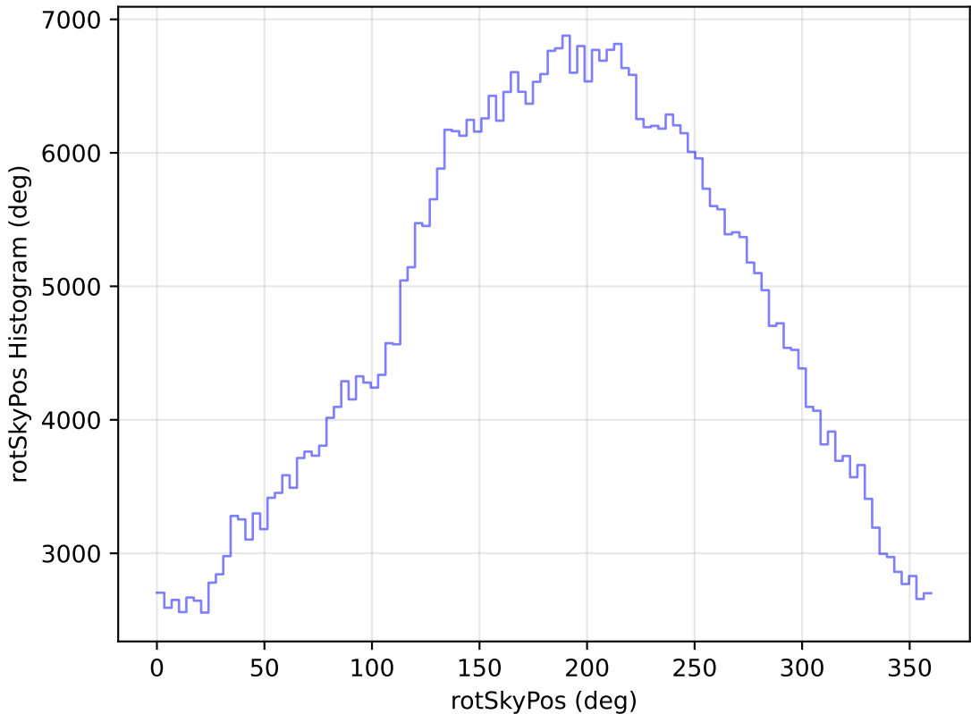
weather_cloudso30v3.4_10yrs WFD r band: rotSkyPos Histogram
