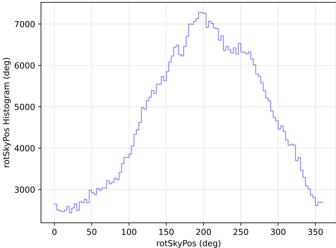
weather_cloudso30v3.4_10yrs WFD i band: rotSkyPos Histogram
