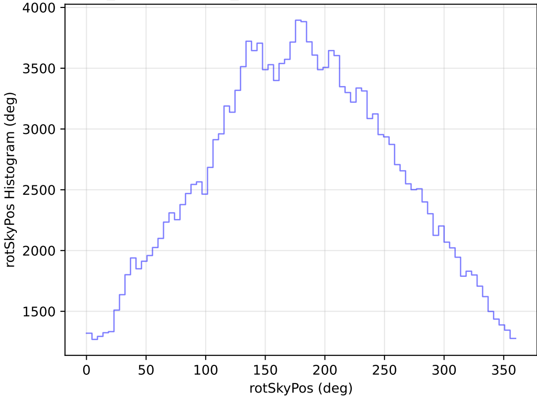
weather_cloudso30v3.4_10yrs WFD g band: rotSkyPos Histogram
