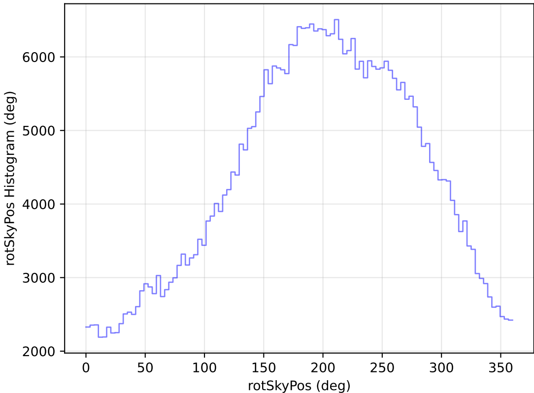
weather_cloudso30v3.4_10yrs All sky z band: rotSkyPos Histogram
