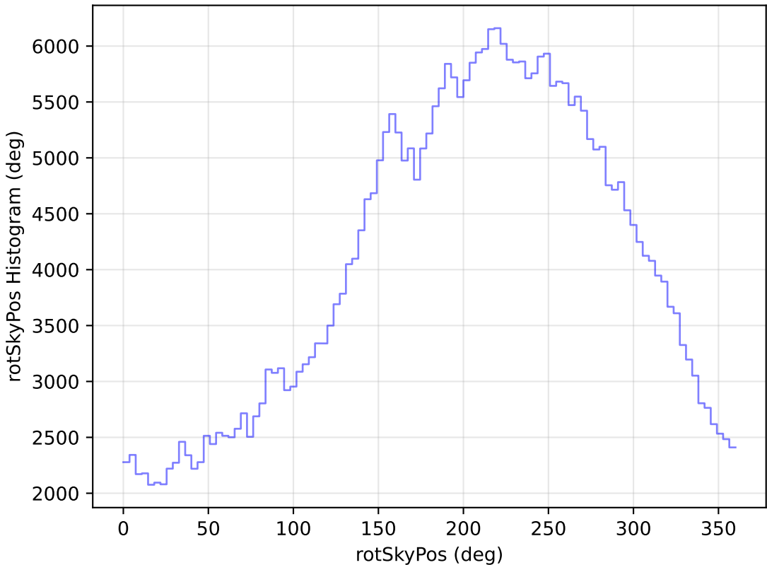
weather_cloudso30v3.4_10yrs All sky y band: rotSkyPos Histogram
