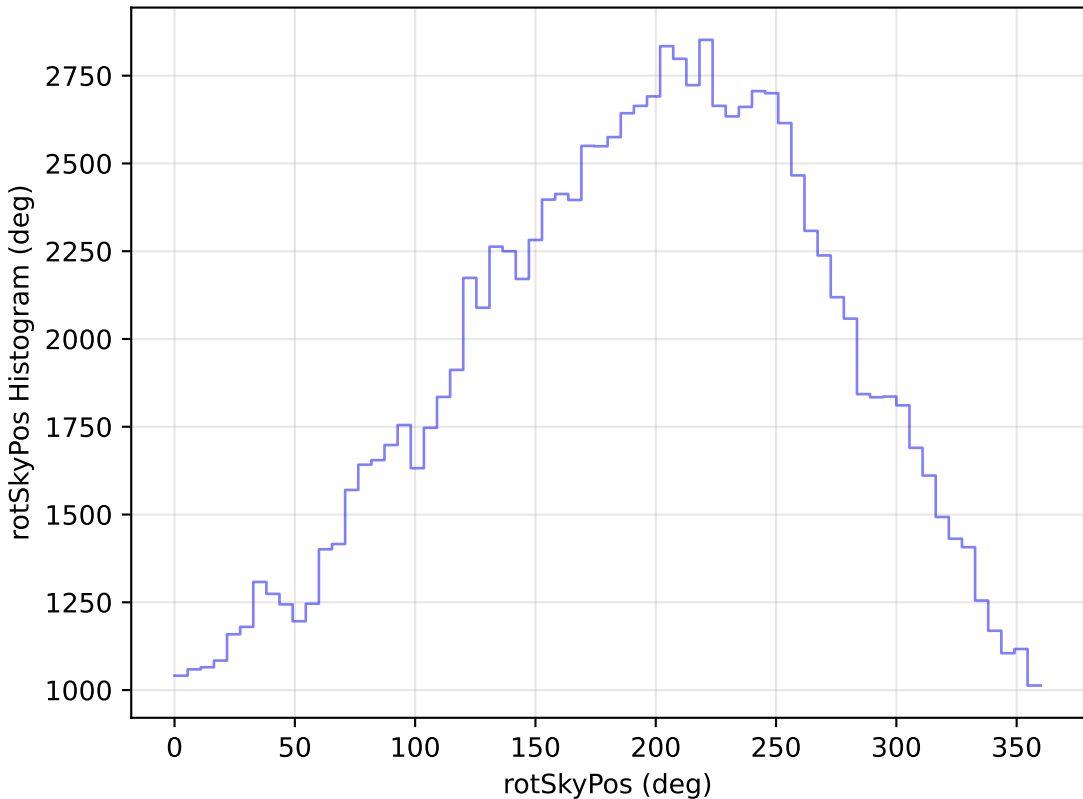
weather_cloudso30v3.4_10yrs All sky u band: rotSkyPos Histogram
