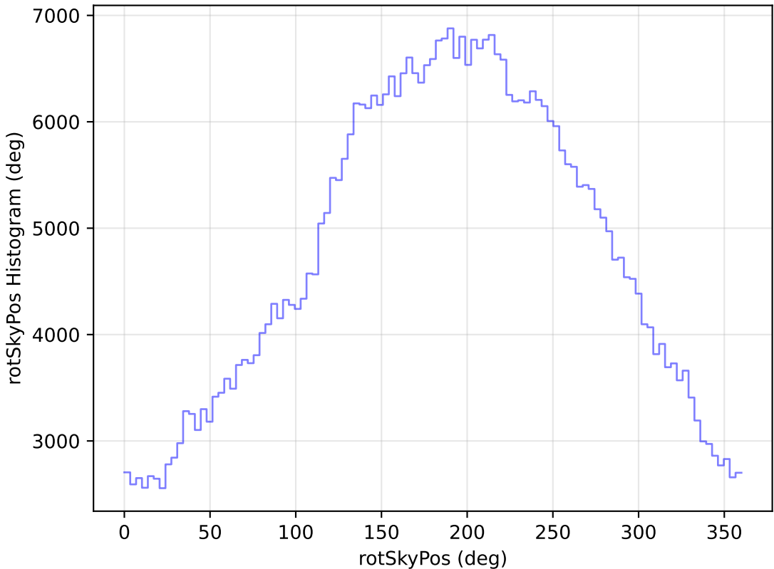
weather_cloudso30v3.4_10yrs All sky r band: rotSkyPos Histogram
