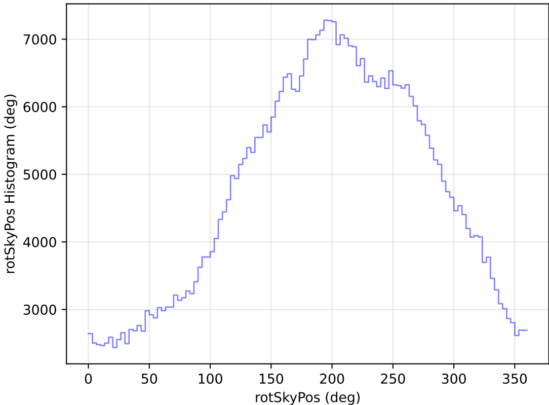
weather_cloudso30v3.4_10yrs All sky i band: rotSkyPos Histogram
