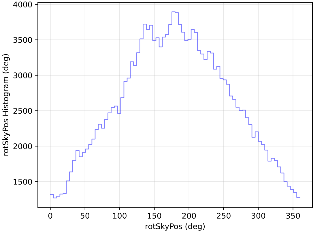
weather_cloudso30v3.4_10yrs All sky g band: rotSkyPos Histogram
