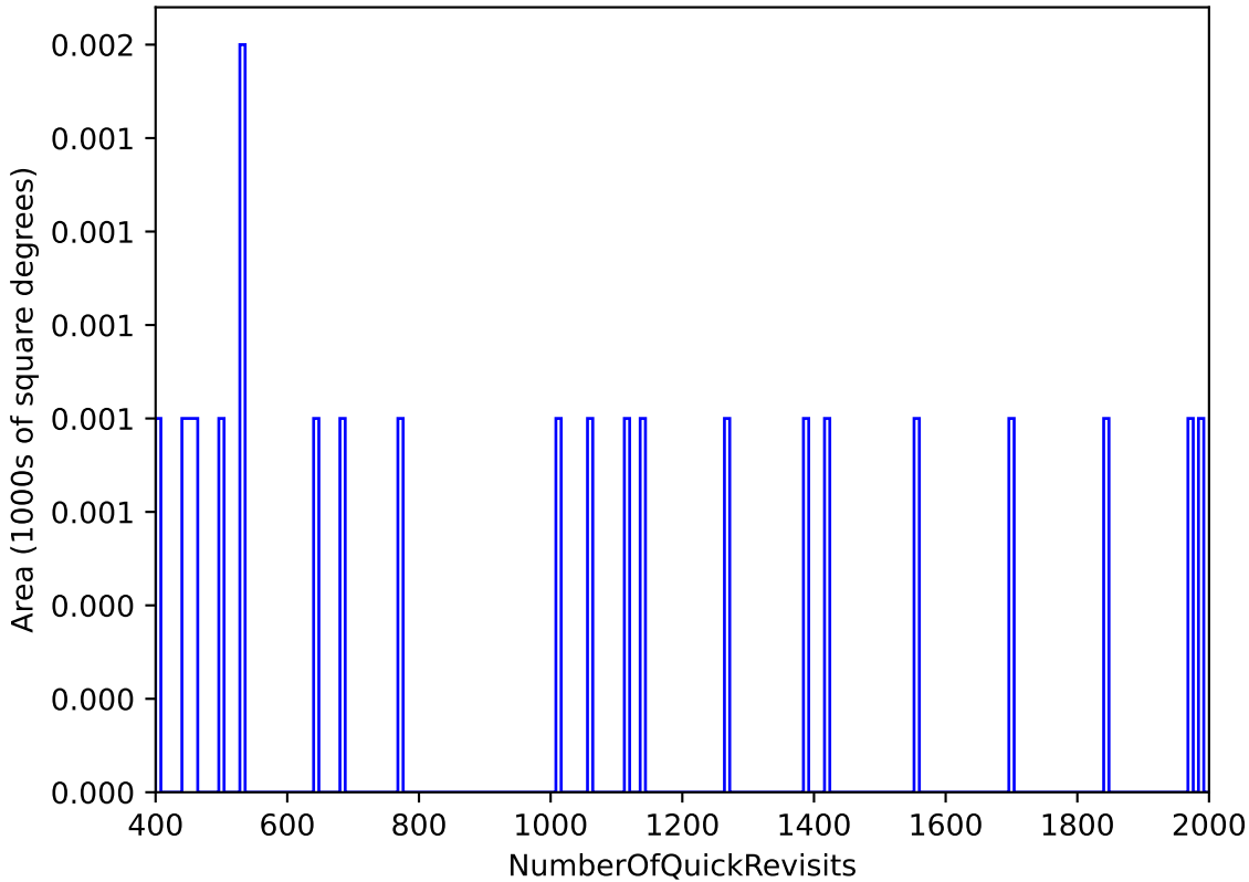
weather_cloudso30v3.4_10yrs All sky: NumberOfQuickRevisits
