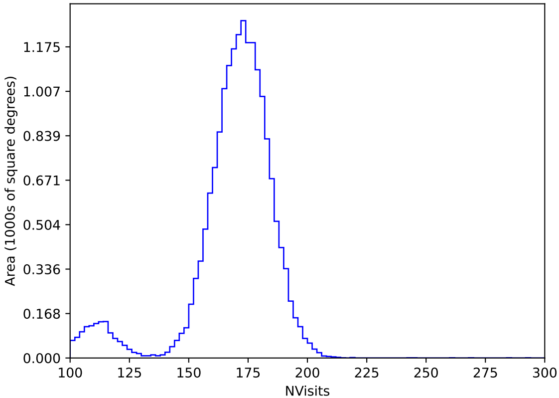
weather_cloudso30v3.4_10yrs WFD y band: NVisits
