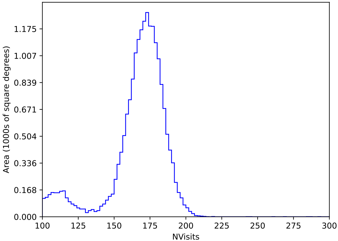
weather_cloudso30v3.4_10yrs All sky y band: NVisits
