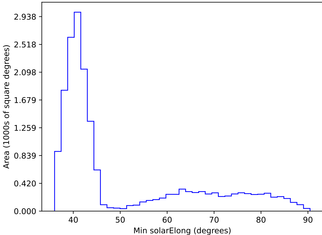
weather_cloudso30v3.4_10yrs WFD i band: Min solarElong
