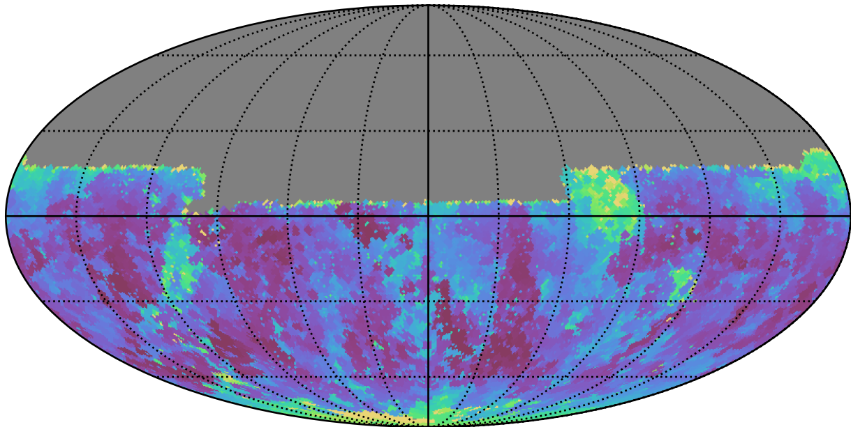
weather_cloudso30v3.4_10yrs Yr 1 y band: Min seeingGeom
