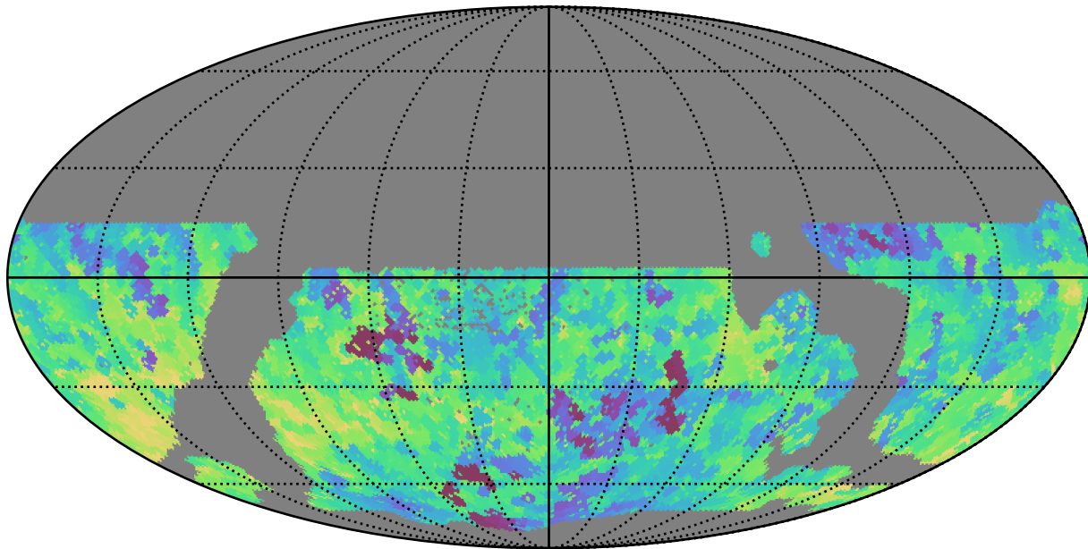
weather_cloudso30v3.4_10yrs WFD z band: Min saturation_mag
