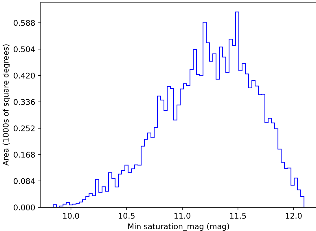
weather_cloudso30v3.4_10yrs WFD u band: Min saturation_mag
