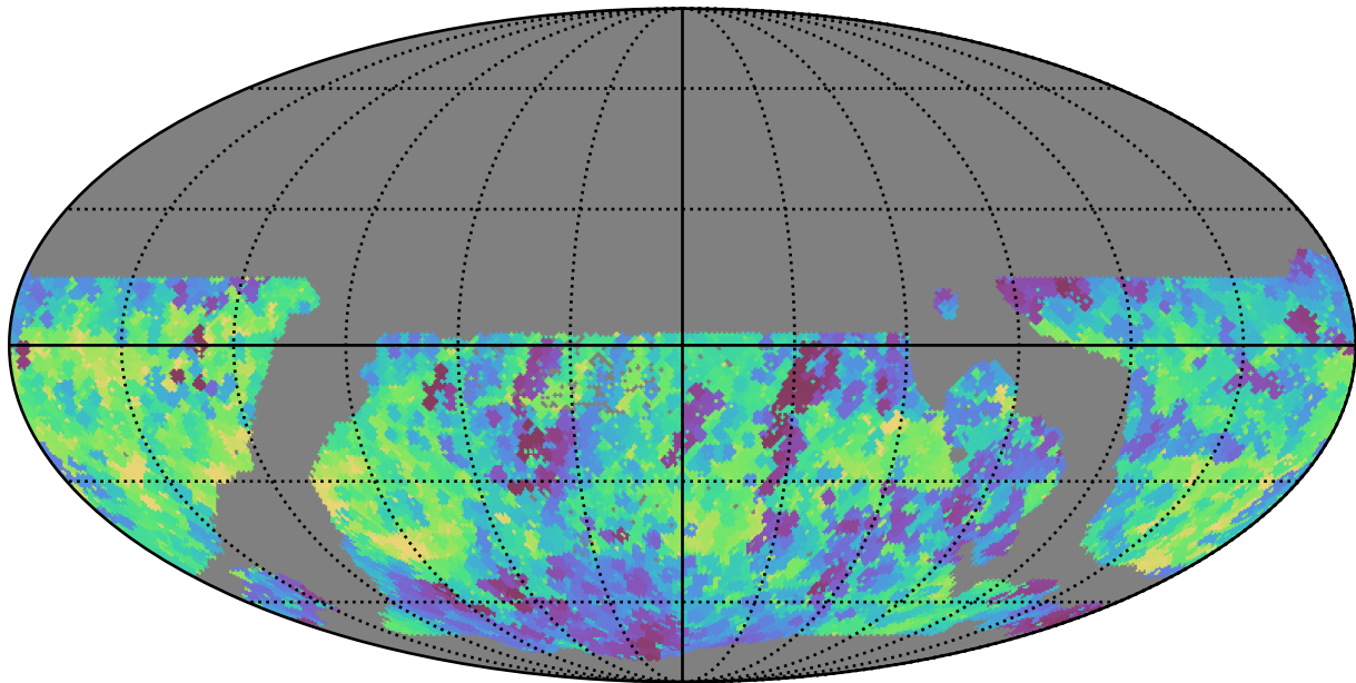
weather_cloudso30v3.4_10yrs WFD r band: Min saturation_mag
