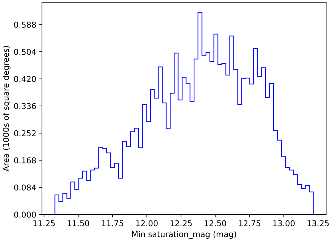
weather_cloudso30v3.4_10yrs WFD r band: Min saturation_mag
