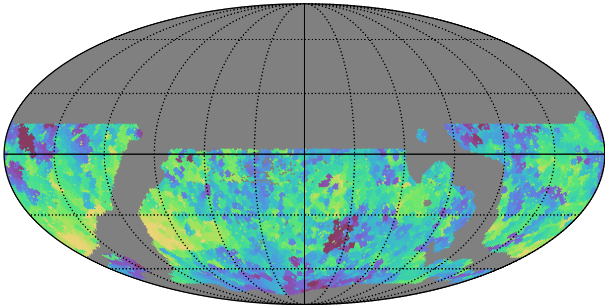
weather_cloudso30v3.4_10yrs WFD i band: Min saturation_mag
