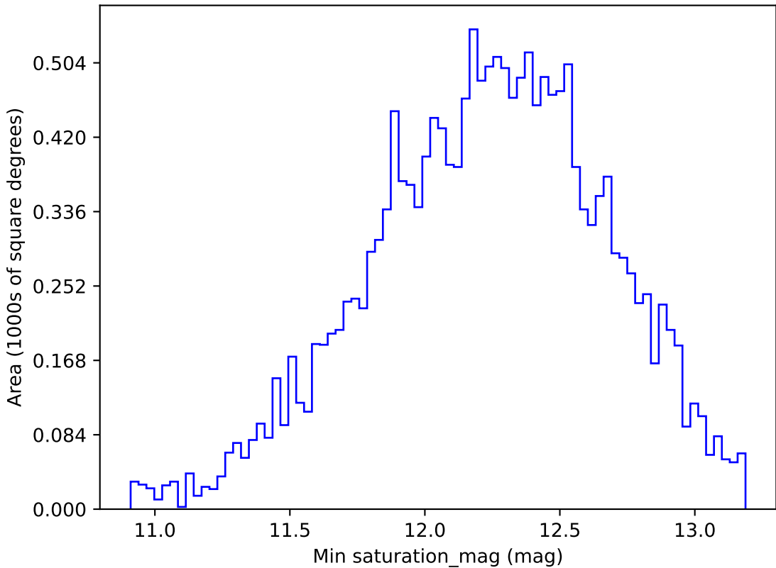
weather_cloudso30v3.4_10yrs WFD i band: Min saturation_mag
