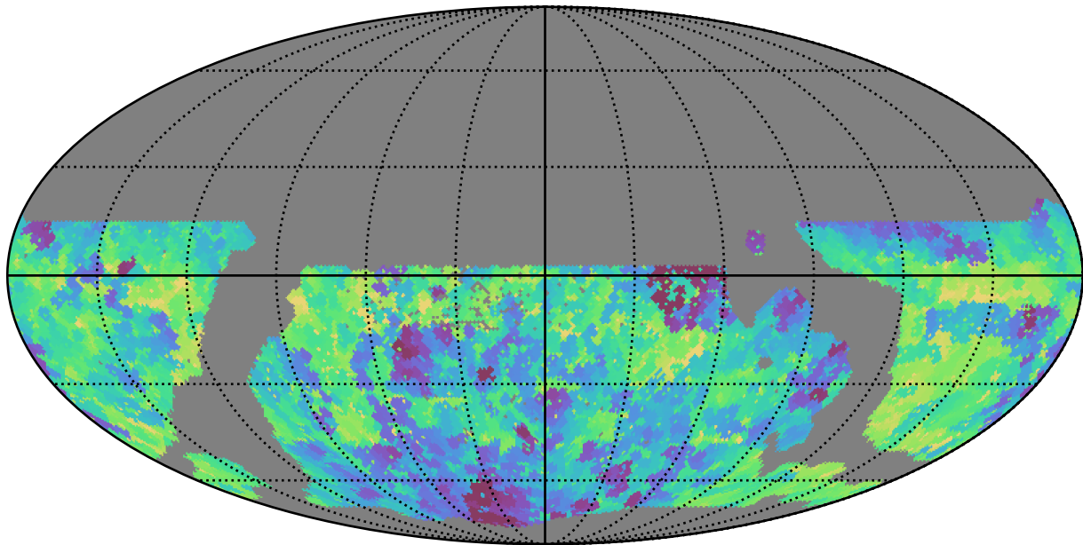
weather_cloudso30v3.4_10yrs WFD g band: Min saturation_mag
