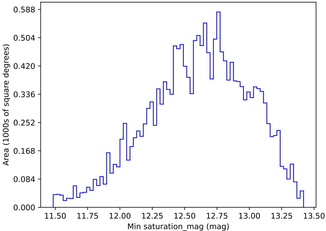
weather_cloudso30v3.4_10yrs WFD g band: Min saturation_mag
