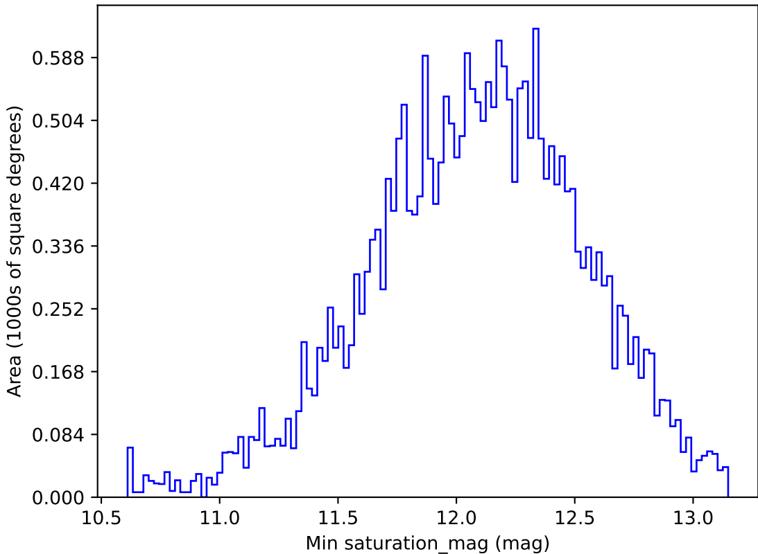
weather_cloudso30v3.4_10yrs All sky z band: Min saturation_mag
