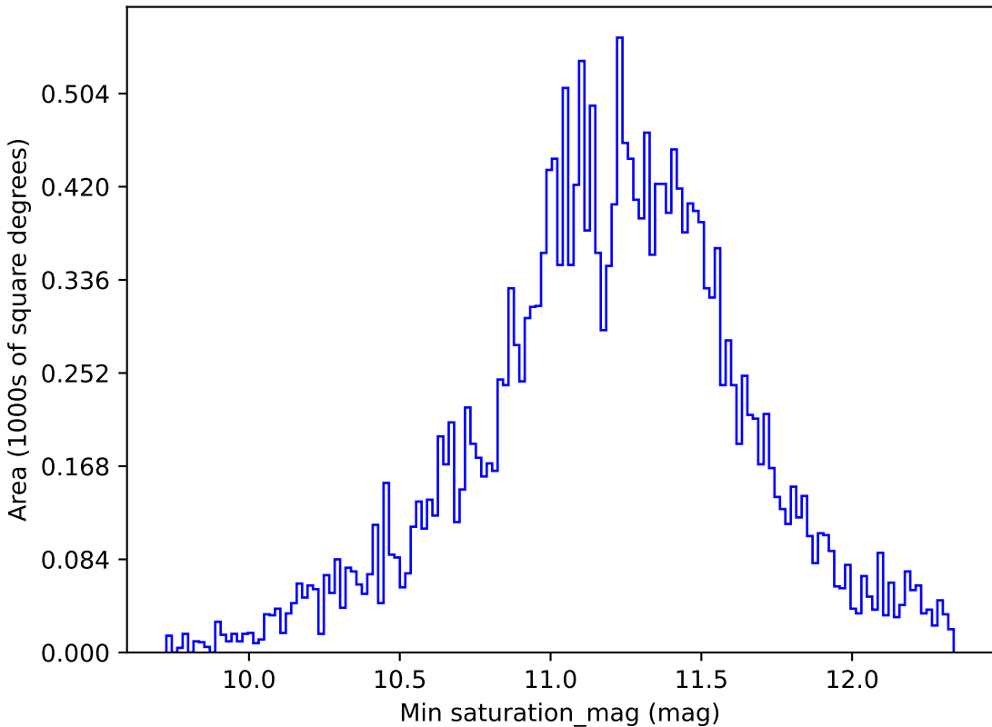
weather_cloudso30v3.4_10yrs All sky y band: Min saturation_mag
