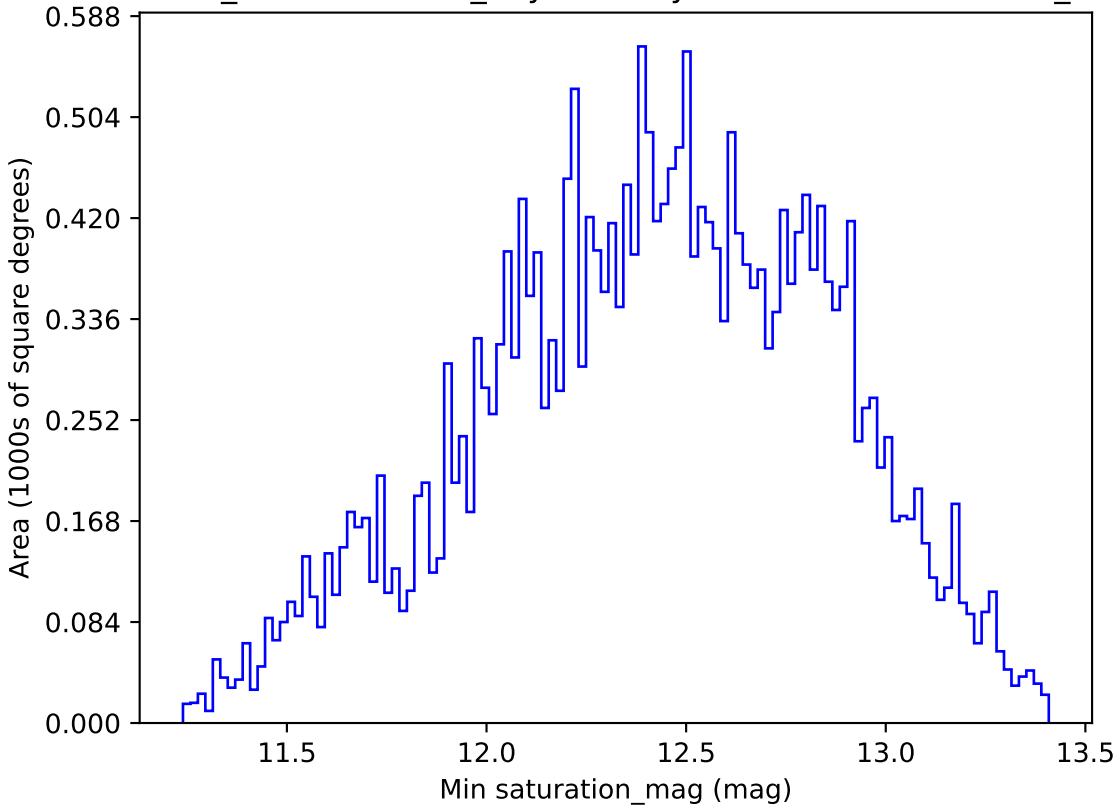
weather_cloudso30v3.4_10yrs All sky r band: Min saturation_mag
