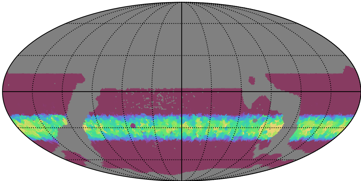
weather_cloudso30v3.4_10yrs WFD y band: Min normairmass
