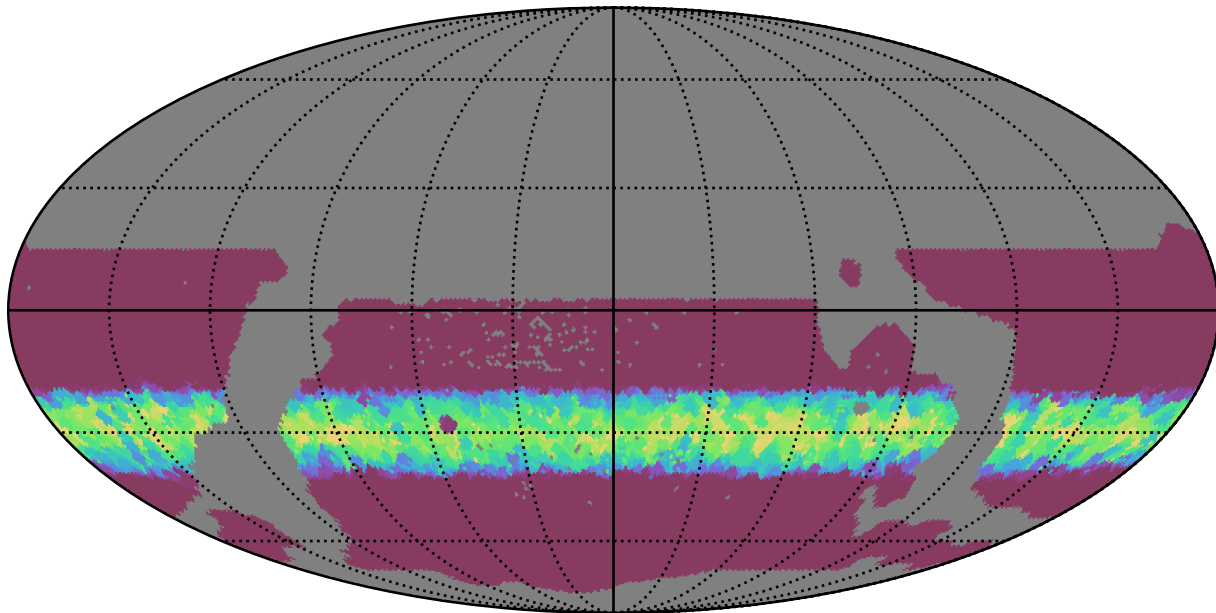
weather_cloudso30v3.4_10yrs WFD i band: Min normairmass
