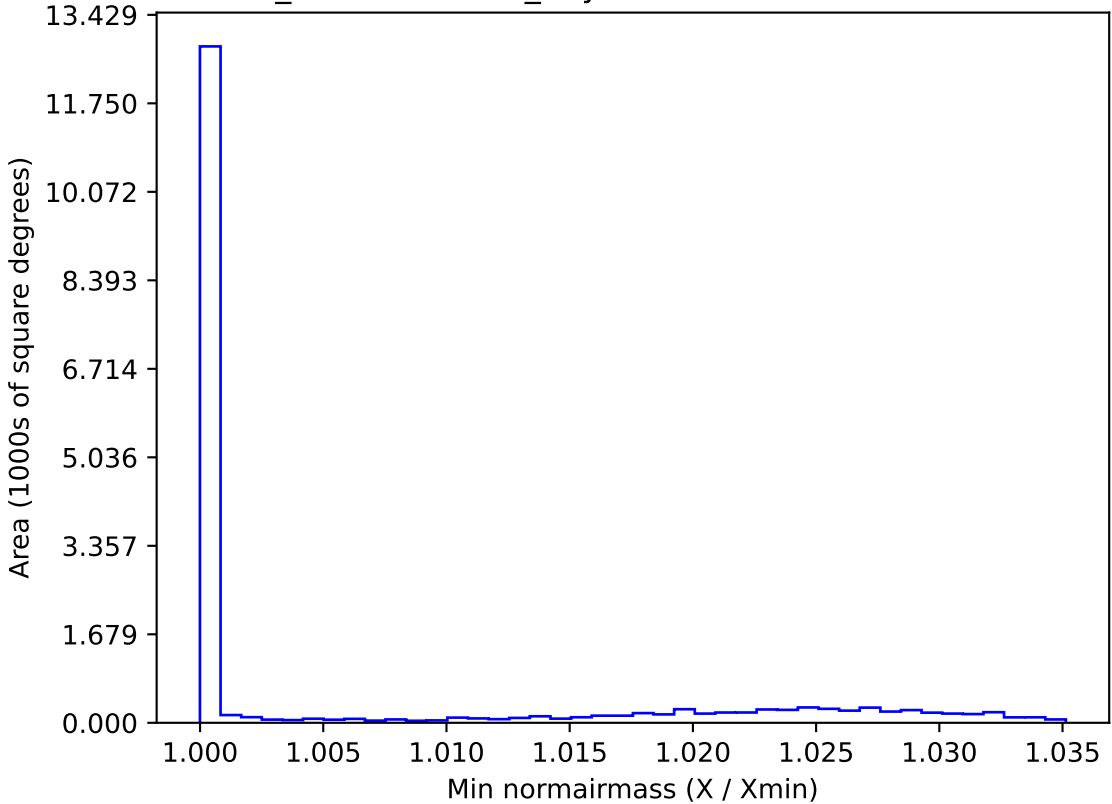
weather_cloudso30v3.4_10yrs WFD i band: Min normairmass
