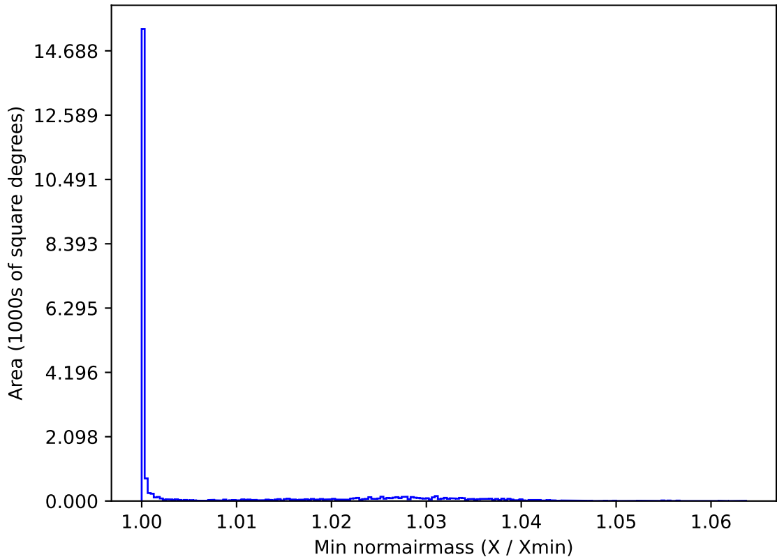
weather_cloudso30v3.4_10yrs All sky y band: Min normairmass
