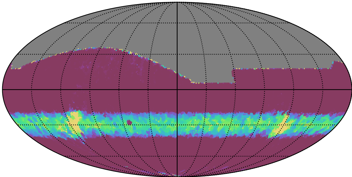
weather_cloudso30v3.4_10yrs All sky i band: Min normairmass
