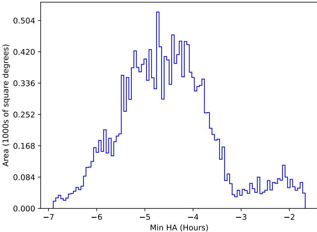
weather_cloudso30v3.4_10yrs WFD z band: Min HA
