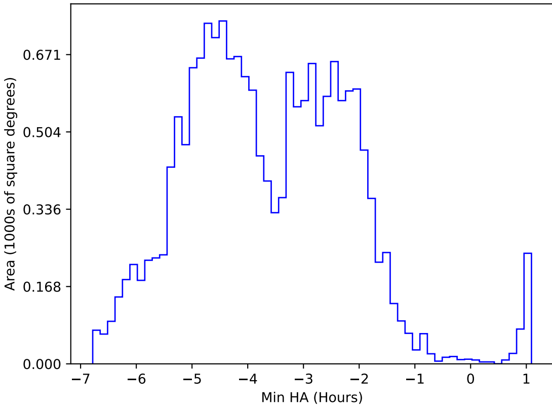
weather_cloudso30v3.4_10yrs WFD y band: Min HA
