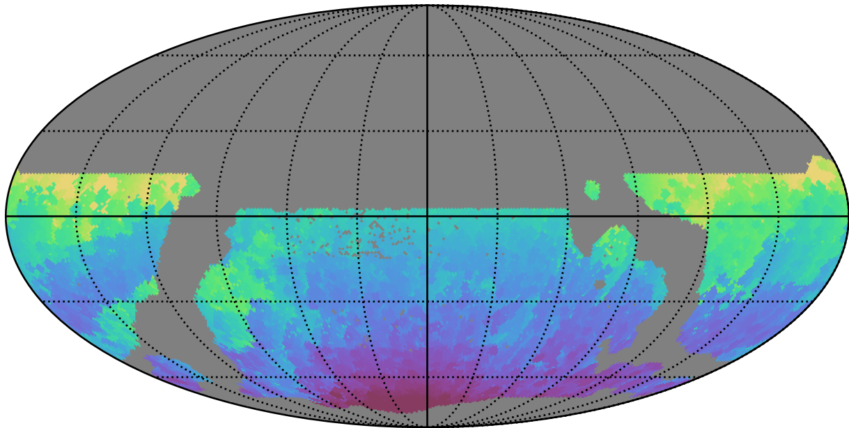
weather_cloudso30v3.4_10yrs WFD i band: Min HA
