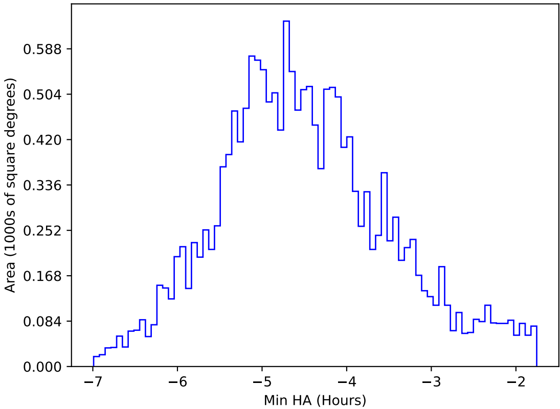
weather_cloudso30v3.4_10yrs WFD i band: Min HA
