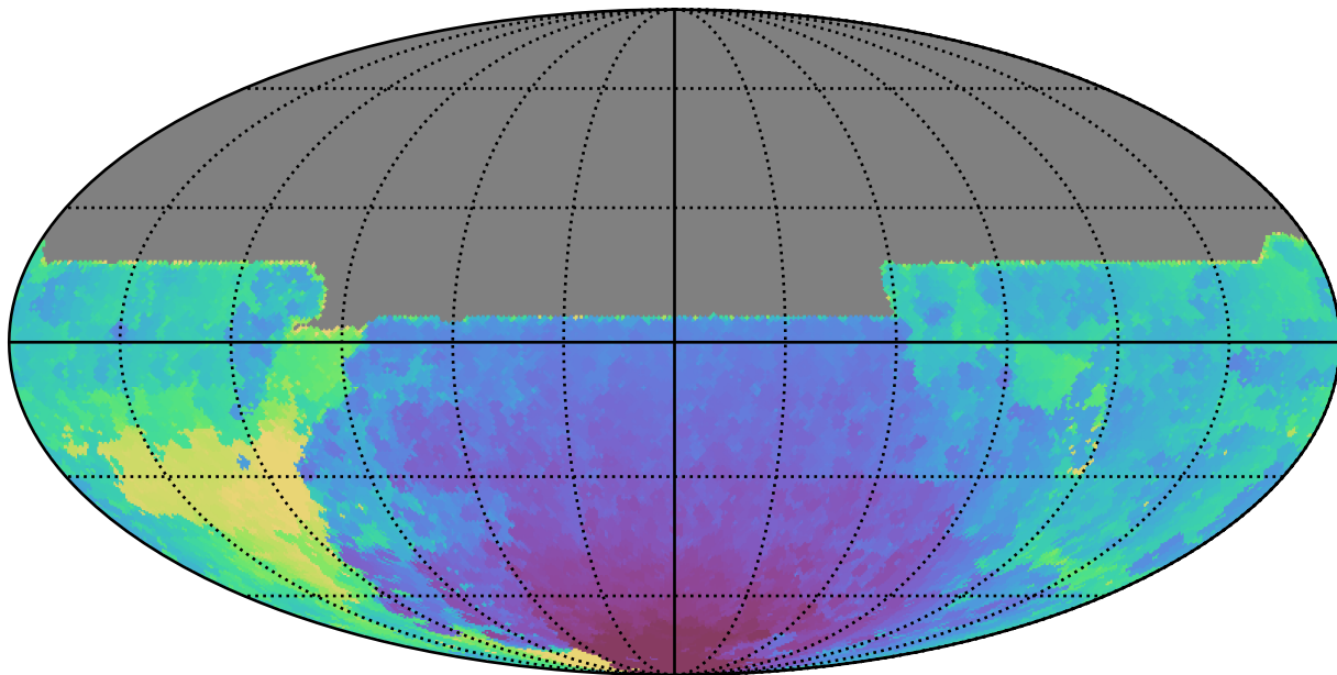
weather_cloudso30v3.4_10yrs All sky y band: Min HA
