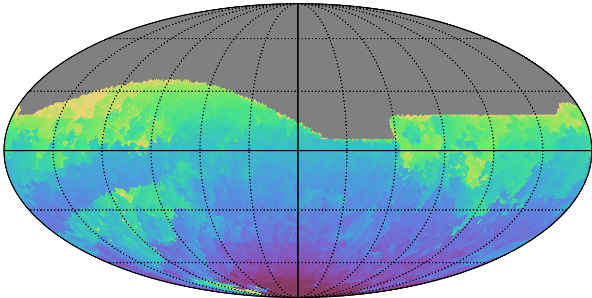
weather_cloudso30v3.4_10yrs All sky i band: Min HA
