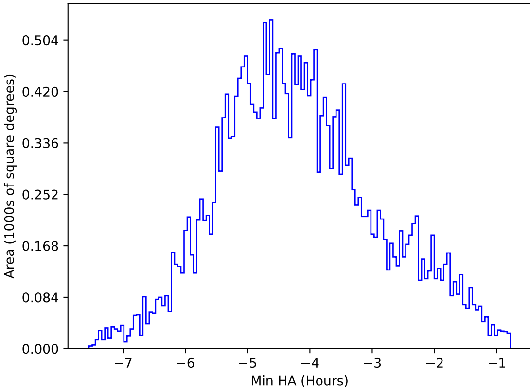
weather_cloudso30v3.4_10yrs All sky i band: Min HA
