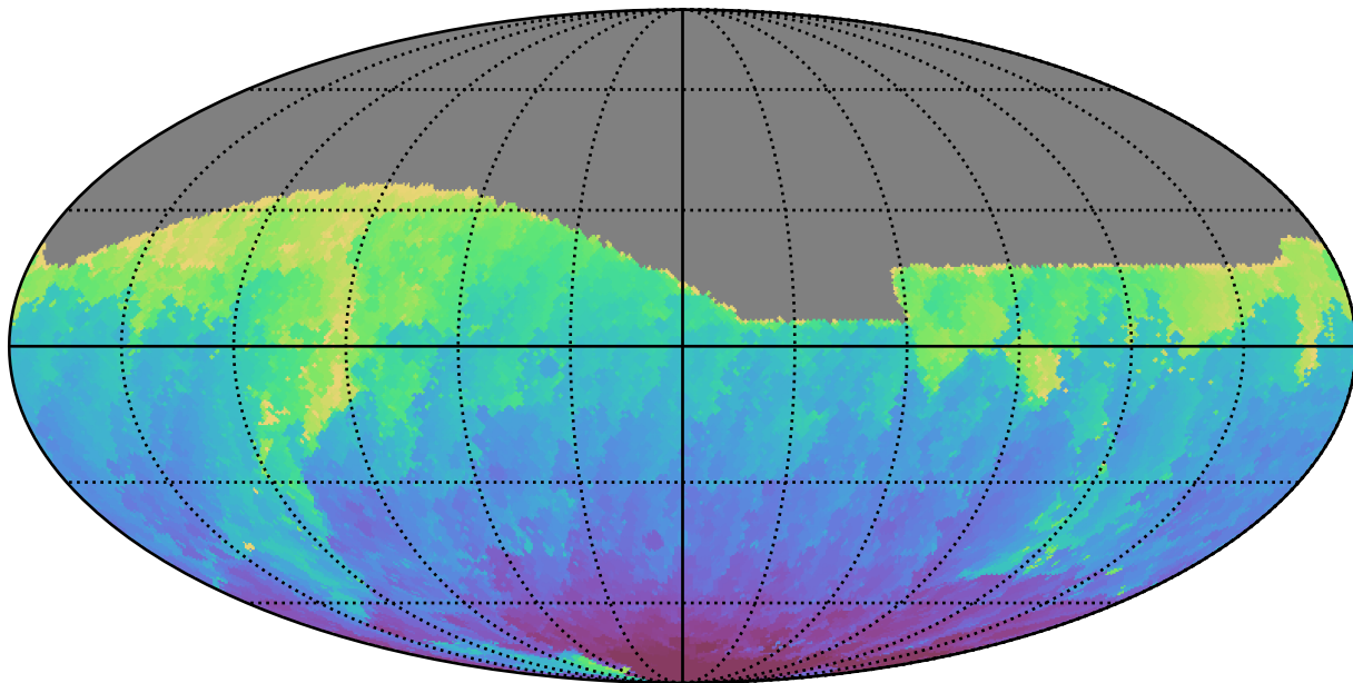
weather_cloudso30v3.4_10yrs All sky g band: Min HA
