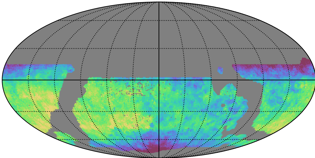
weather_cloudso30v3.4_10yrs WFD y band: Median saturation_mag
