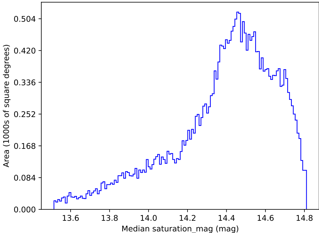
weather_cloudso30v3.4_10yrs All sky i band: Median saturation_mag
