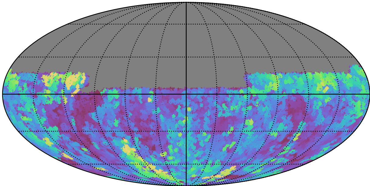
weather_cloudso30v3.4_10yrs Yr 1 y band: Max seeingGeom
