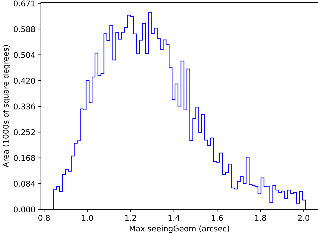
weather_cloudso30v3.4_10yrs Yr 1 y band: Max seeingGeom
