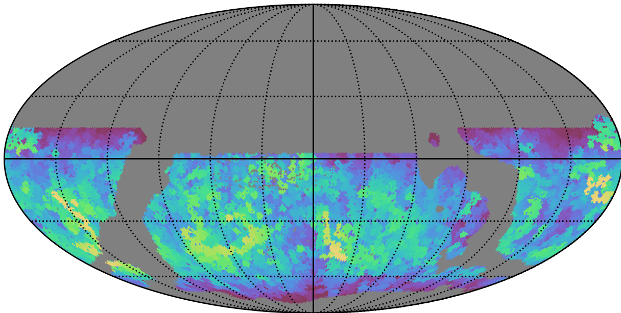
weather_cloudso30v3.4_10yrs WFD y band: Max saturation_mag
