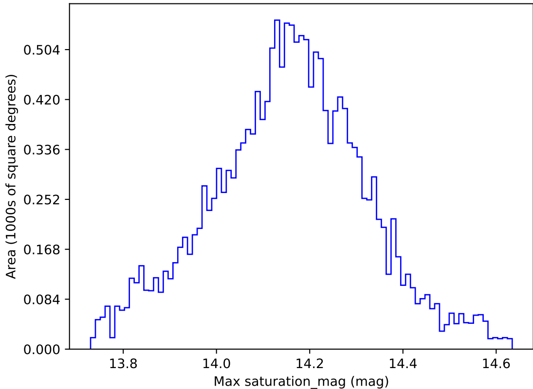
weather_cloudso30v3.4_10yrs WFD y band: Max saturation_mag
