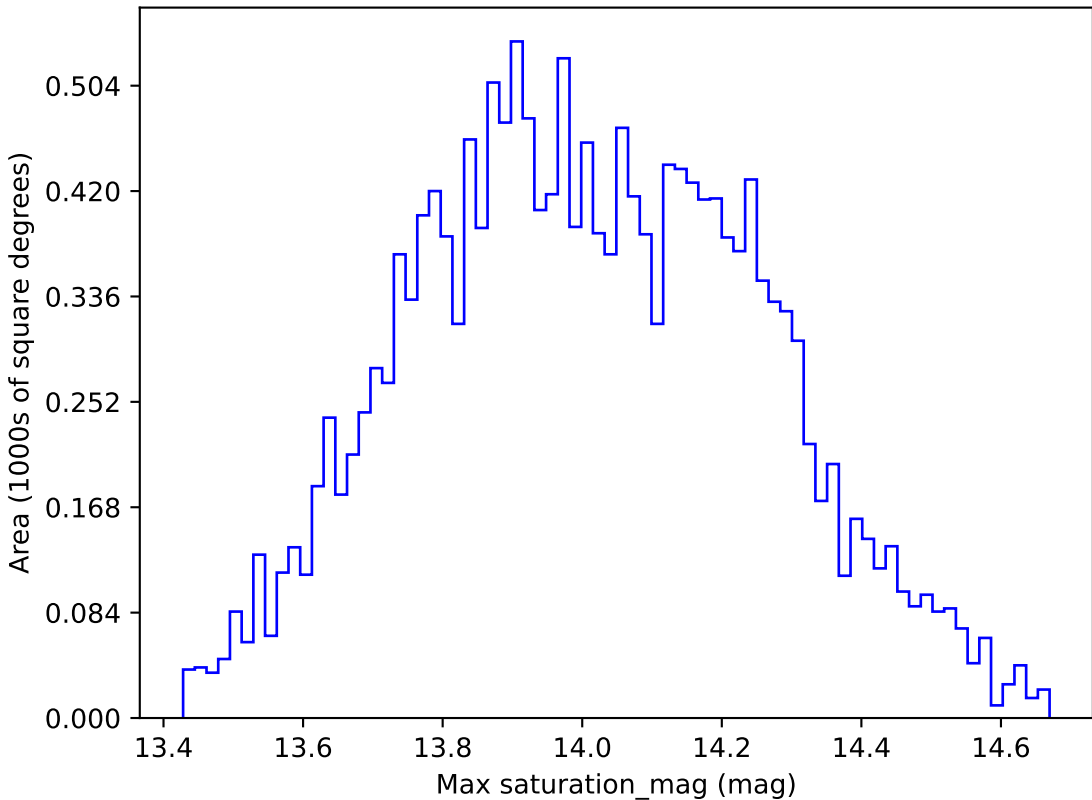
weather_cloudso30v3.4_10yrs WFD u band: Max saturation_mag
