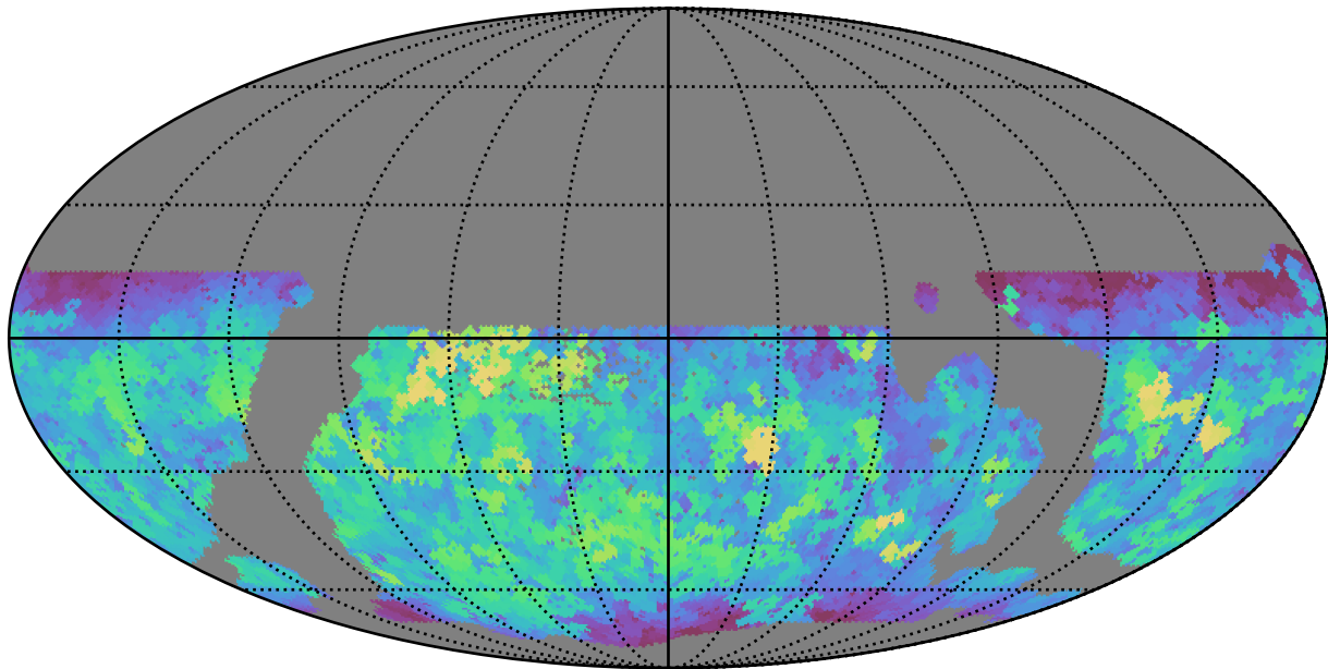
weather_cloudso30v3.4_10yrs WFD r band: Max saturation_mag
