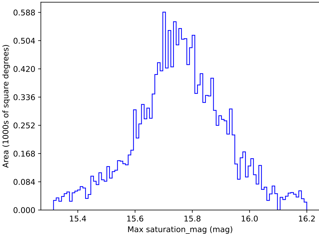
weather_cloudso30v3.4_10yrs WFD r band: Max saturation_mag
