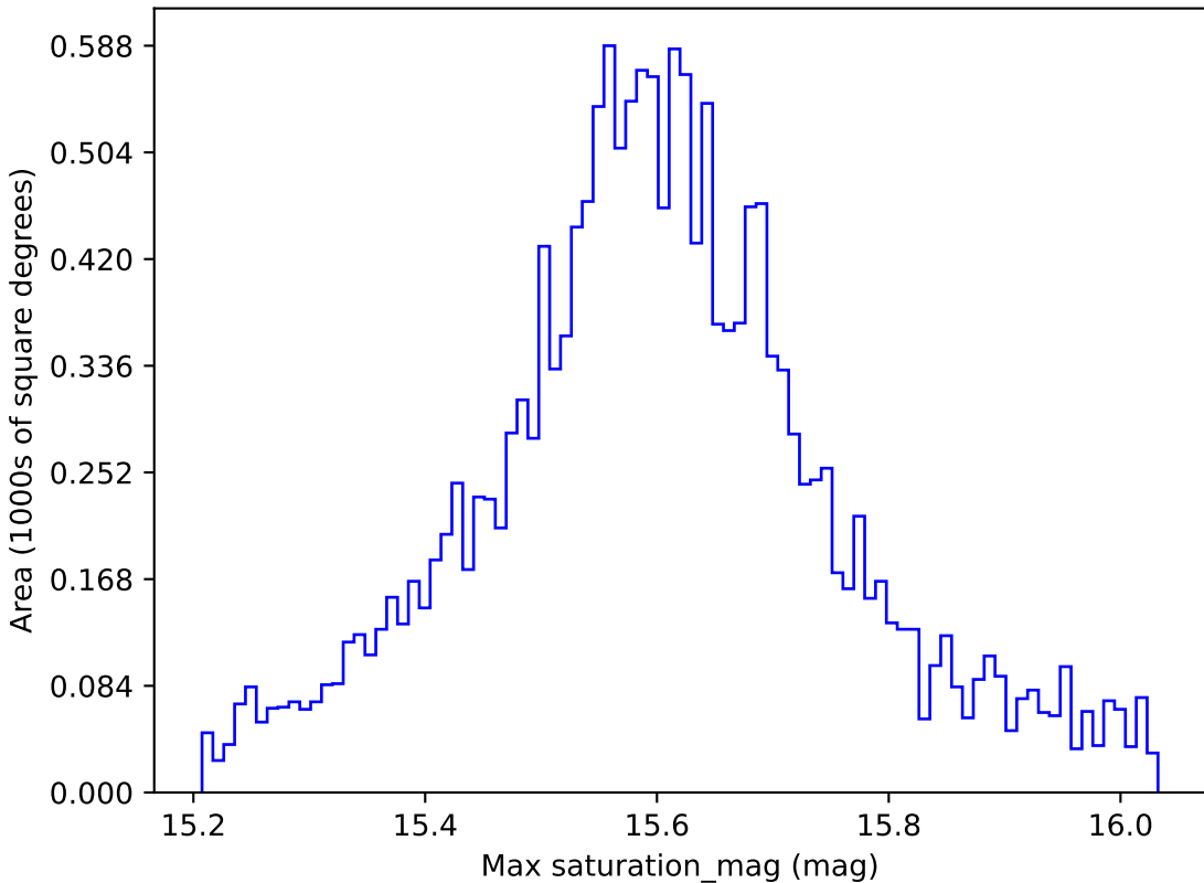
weather_cloudso30v3.4_10yrs WFD i band: Max saturation_mag
