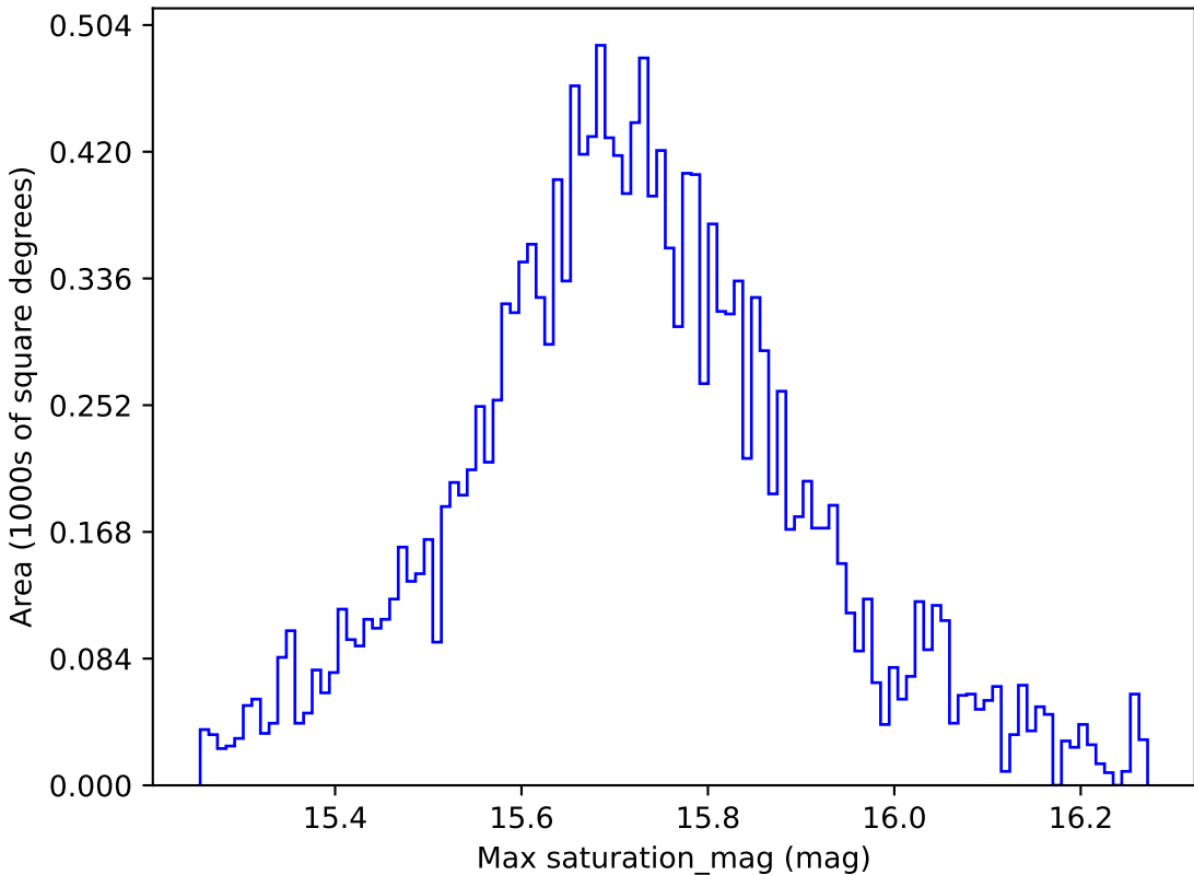
weather_cloudso30v3.4_10yrs WFD g band: Max saturation_mag
