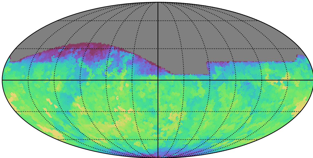
weather_cloudso30v3.4_10yrs All sky z band: Max saturation_mag
